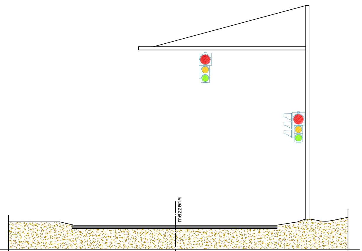
VISTA B-B' (direzione Sassuolo) - scala 1:50
