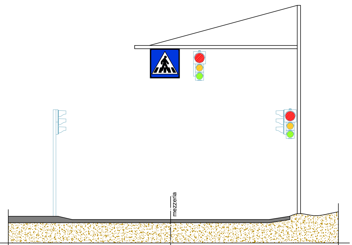
VISTA A-A' (direzione Rubiera) - scala 1:50
