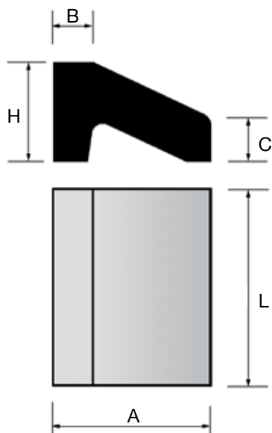
CORDOLO SPARTITRAFFICO
