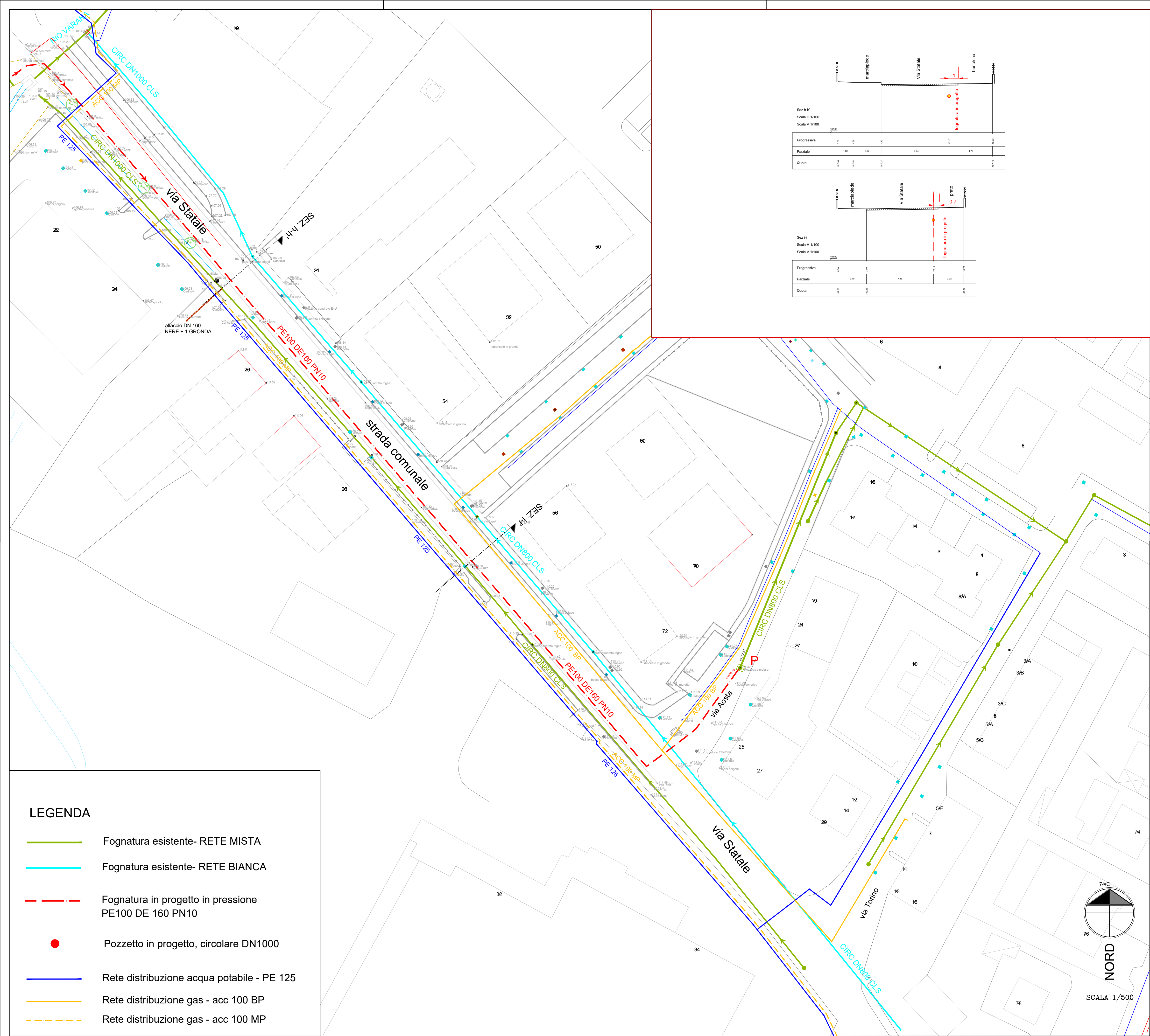
PLANIMETRIA DI PROGETTO - scala 1:500
