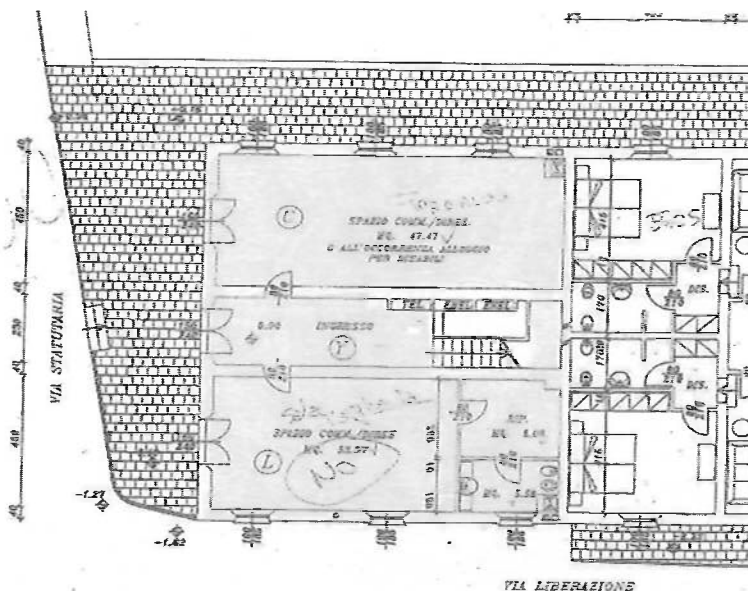
PIANTA PIANO RIALZATO
